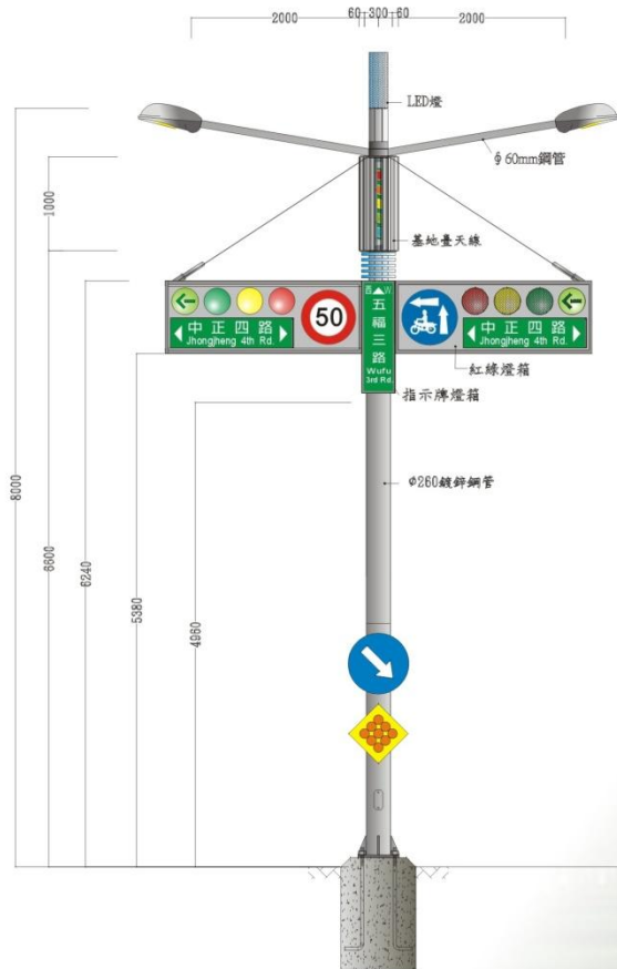
正向立面圖 FRONT ELEVATION
