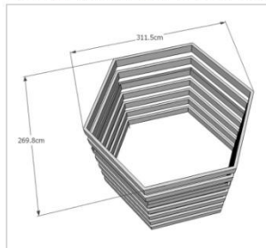
基地台尺寸圖
