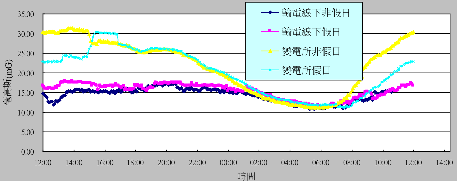
變電所及輸電線下二十四小時連續監測
