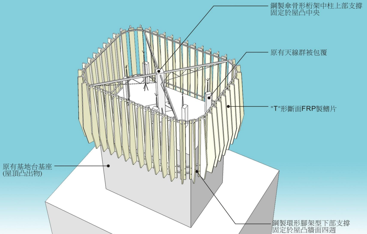
2009 基地台美化創意設計比賽 3D俯視圖
