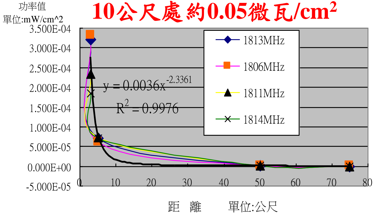
圖三. 電磁波功率密度值與距離關係
